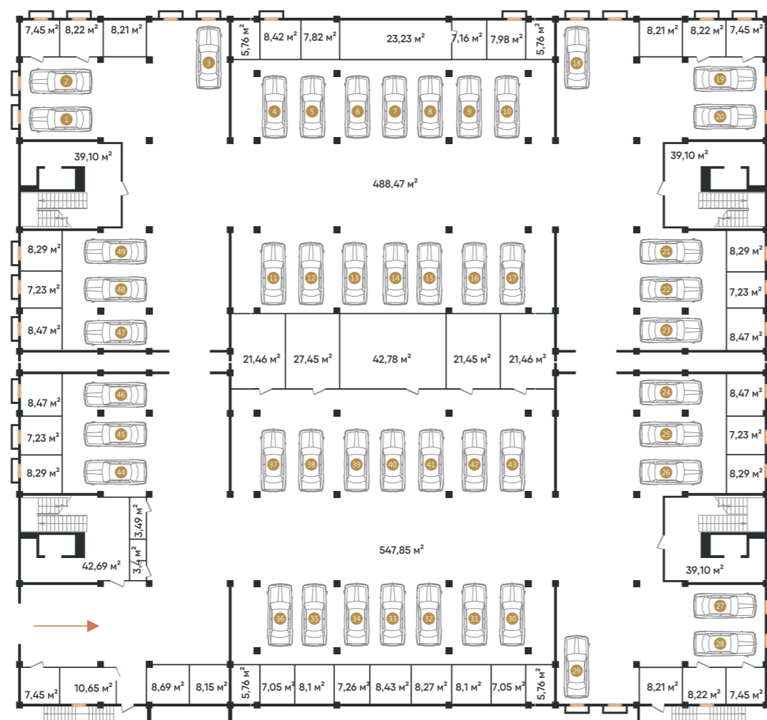
План подземного паркинга | 3-4 блоки
